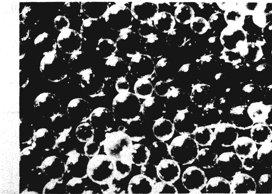
Fig. 5. Copoly(styrene-1%-divinylbenzene) resin.
